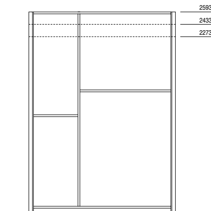
Altezze moduli senza ante Height modules without doors
