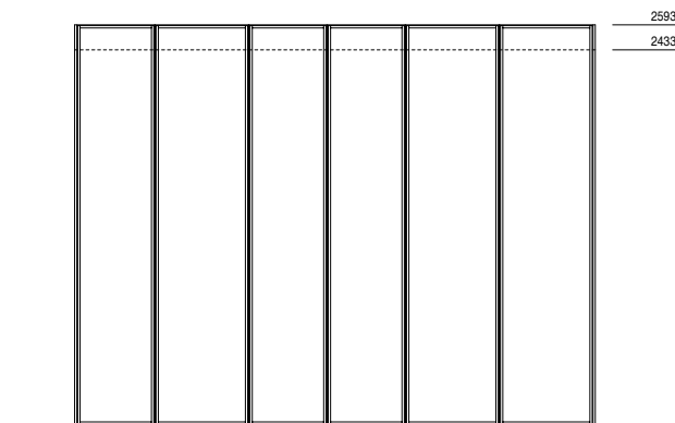
Altezze moduli con ante Heights modules with doors
